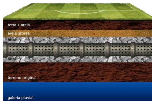
Figura 4: Imagem esquemática do sistema de drenagem. Fonte: Acervo Caetés.
